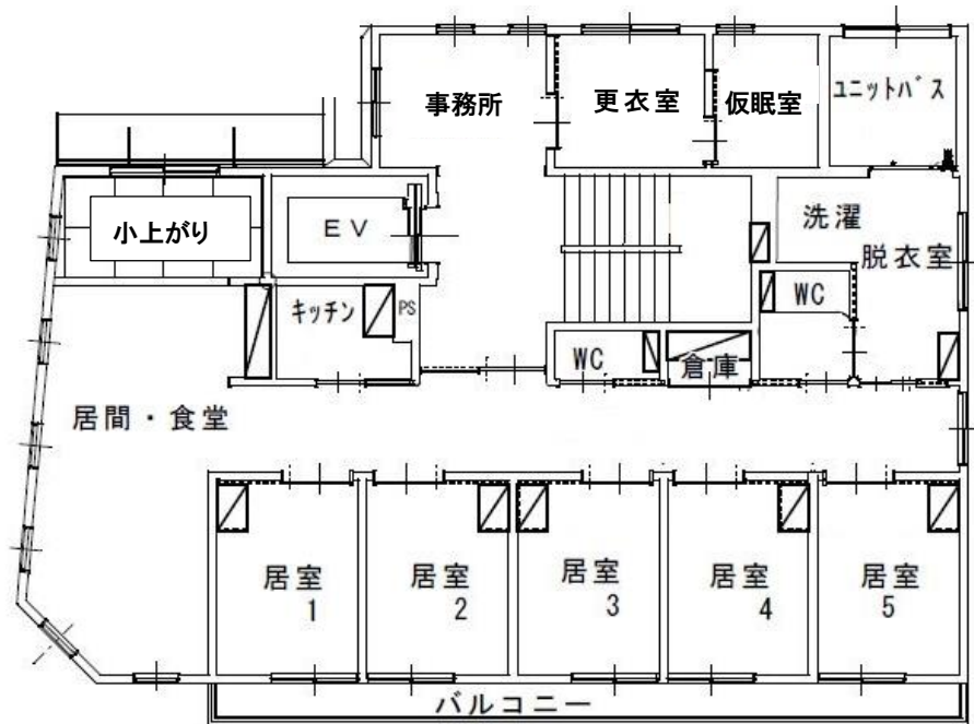
1階平面図
